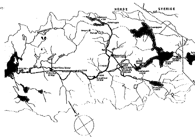
Oversikt over kraftverk, overføringer, demninger og magasiner i Selbu og Tydal.
