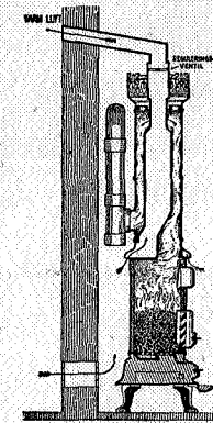
„REKORD“ opvarmer et tilstøtende værelse
