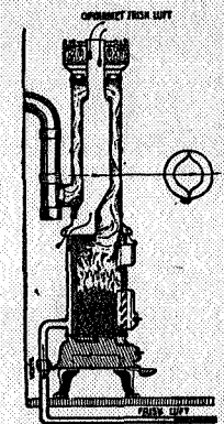
„REKORD“ med Friskluftsledning
