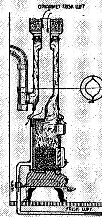
„RECORD“ med Friskluftsledning
