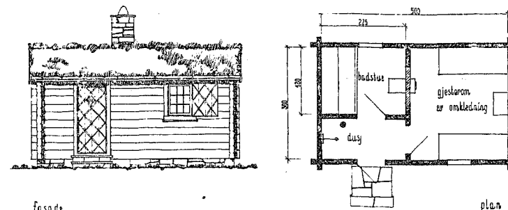
fasade
