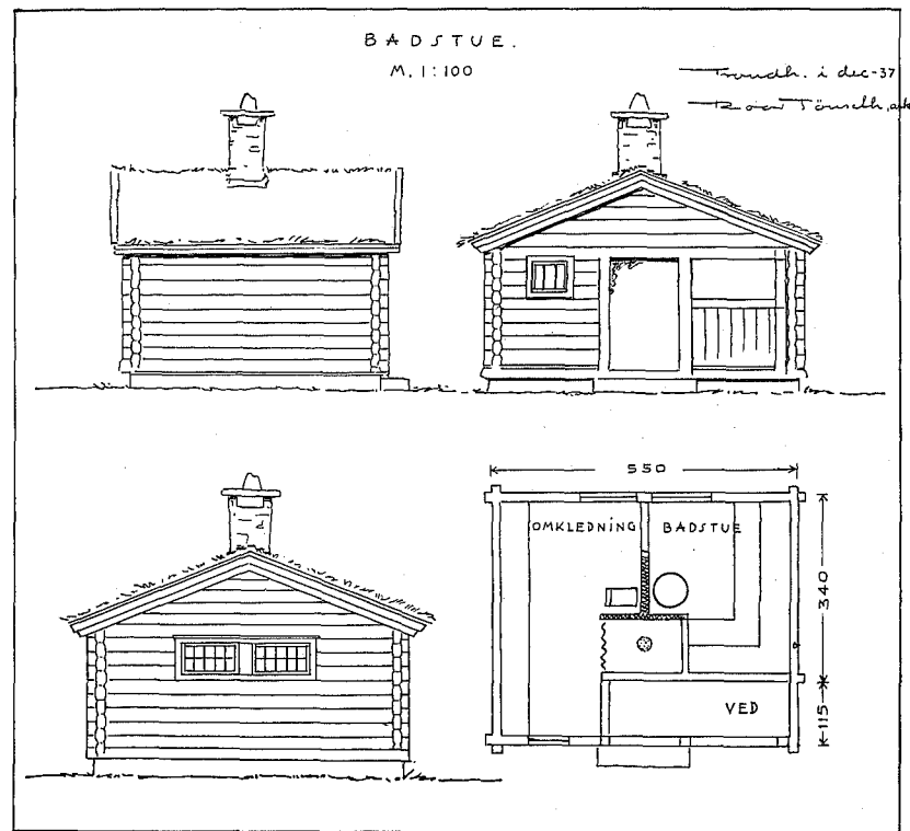
Riss av badstuen på Nedalen.
